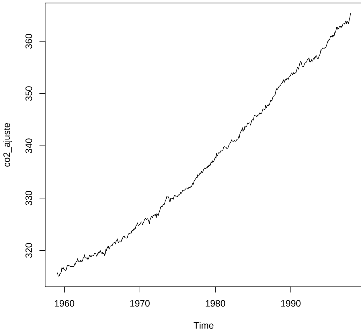
Serie CO2 ajustee (CVS)
